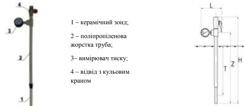
Рисунок 1 Тензіометр вологості ґрунту іригаційний Акватек
